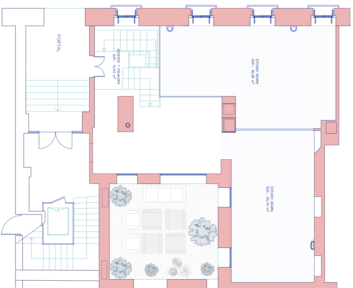
PLANTA BAJA SUP. UTIL: 91,02 m 2 SUP. CONSTRUIDA: 115,41 m 2
